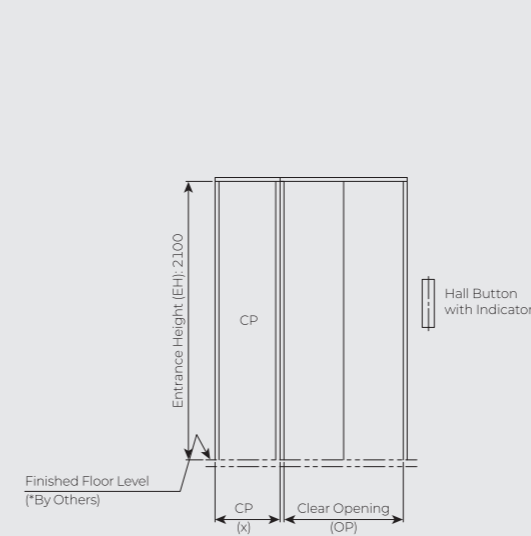
WE050 TYPE (STANDARD)
