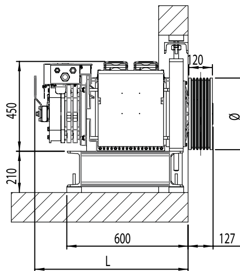
SEZIONE A-A
